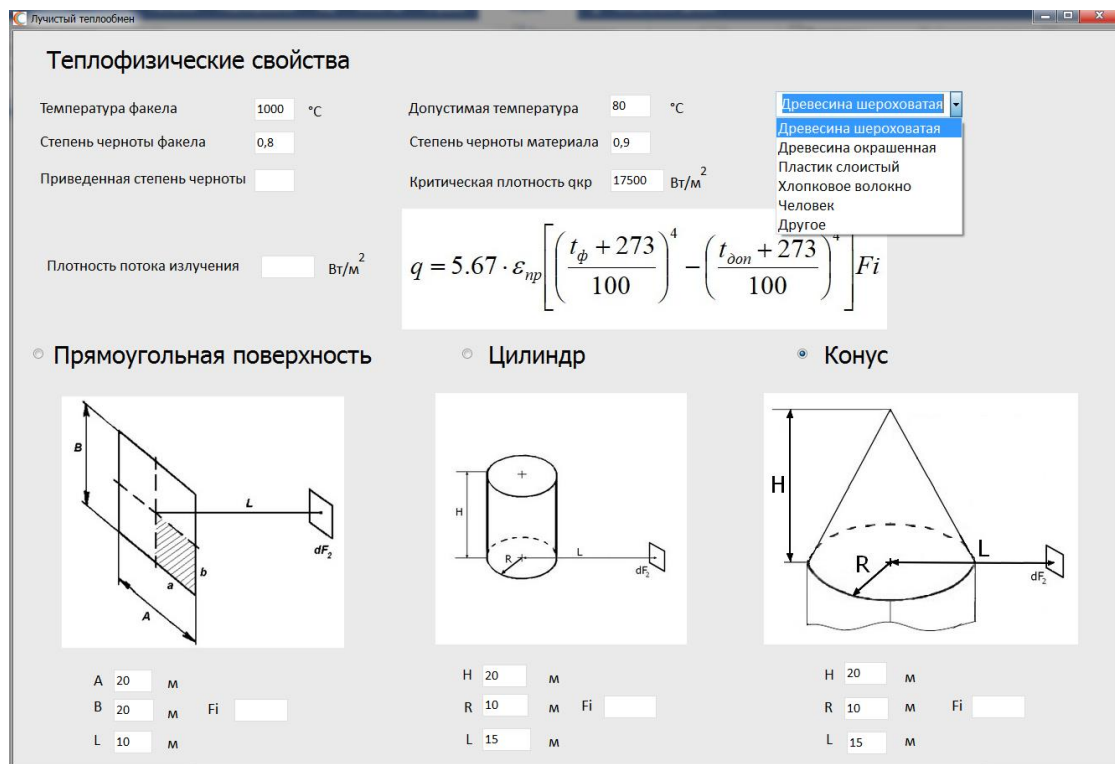
Рис. 4. Рабочее окно программы
