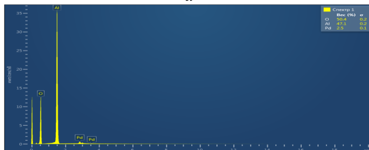
Рис. 5. Качественный (а) и количественный (б) химический состав и распределение частиц каталитической фракции по поверхности сорбционного носителя в условиях предварительной пропитки 40% дистиллированной водой от максимального впитывания (увеличение 500 раз)
