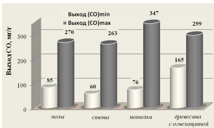
Рис. 1. Минимальные и максимальные значения удельных выходов оксида углерода (СО), зафиксированные при горении материалов на основе древесины и ее заменителей, используемых при различных вариантах отделки
