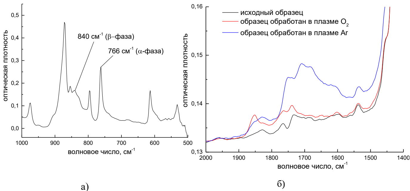
Рис. 1. ИК спектр НПВО пленки ПВДФ
