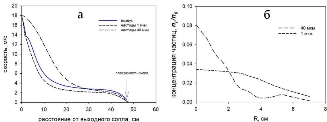
Рис. 2. а) Зависимость скорости от расстояния до выходного сопла (поверхность очага на расстоянии 47 см);
