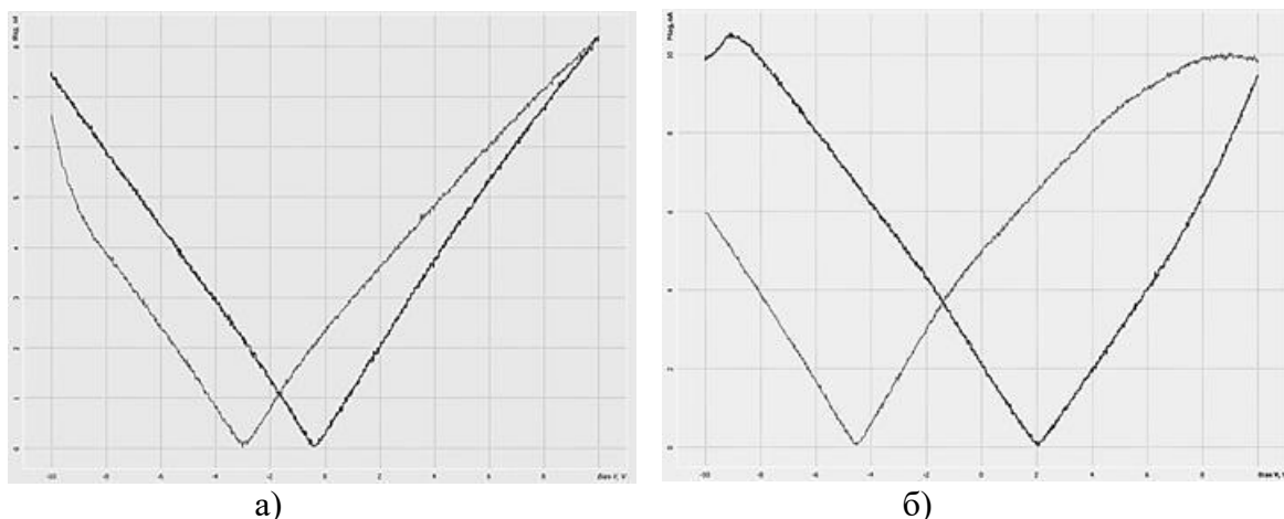
Рис. 4. Амплитудные кривые СМП спектроскопии:
