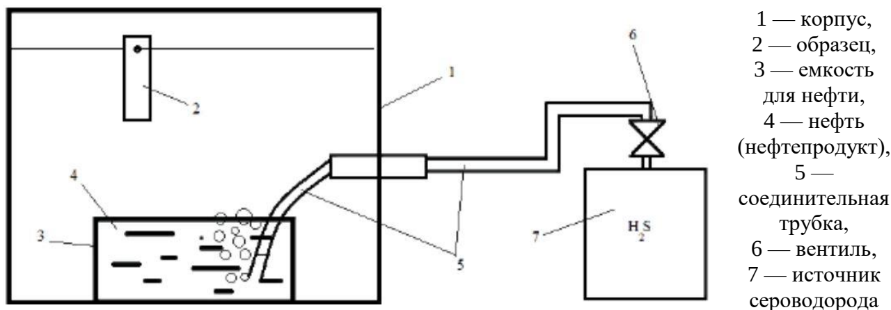
Рис. 1. Принципиальная схема лабораторной установки, имитирующей условия паровоздушного пространства в резервуаре для хранения нефти и нефтепродуктов
