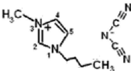
Рис. 1. Структура катиона 1-бутил-3-метилимидазолия и дицианамид-аниона
