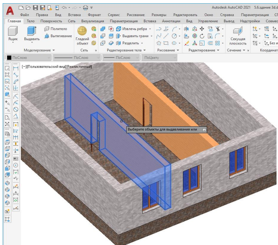
Рис. 3. Трехмерная модель первого этажа здания, выполненная на основе чертежа плана здания
