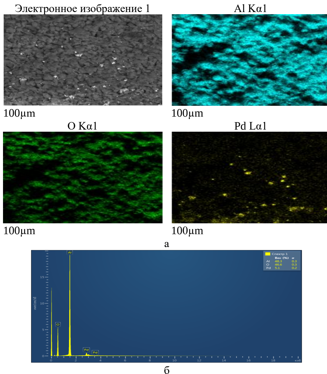
Рис. 11. Качественный и количественный химический состав и распределение частиц каталитической фракции по поверхности сорбционного носителя в условиях предварительной пропитки 80% дистиллированной водой от максимального впитывания (увеличение 500 раз)
